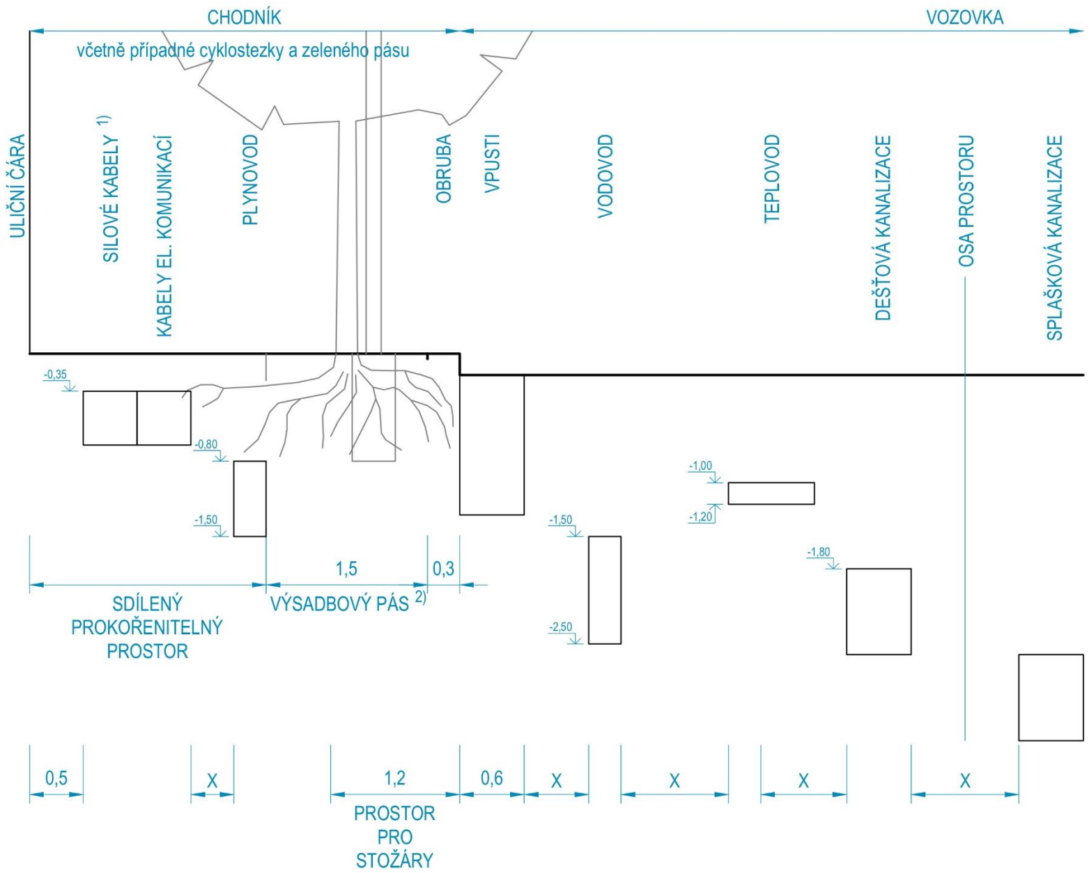
Obr C.2 - Zájmová pásma jednotlivých druhů vedení technického vybavení v uličním prostranství a jejich posloupnost při stanovení výsadbového pásu v chodníku
