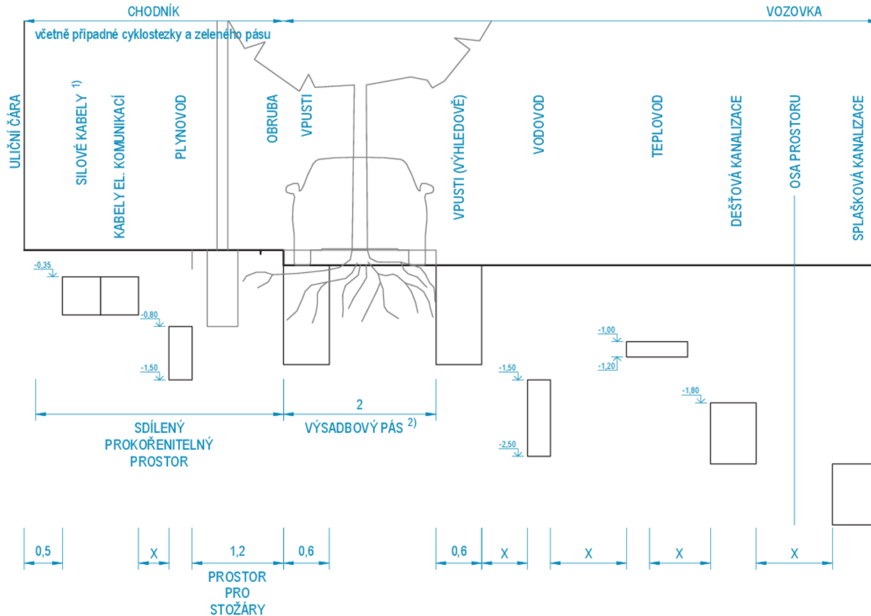
Obr C.3 - Zájmová pásma jednotlivých druhů vedení technického vybavení v uličním prostranství a jejich posloupnost při stanovení výsadbového pásu ve vozovce
